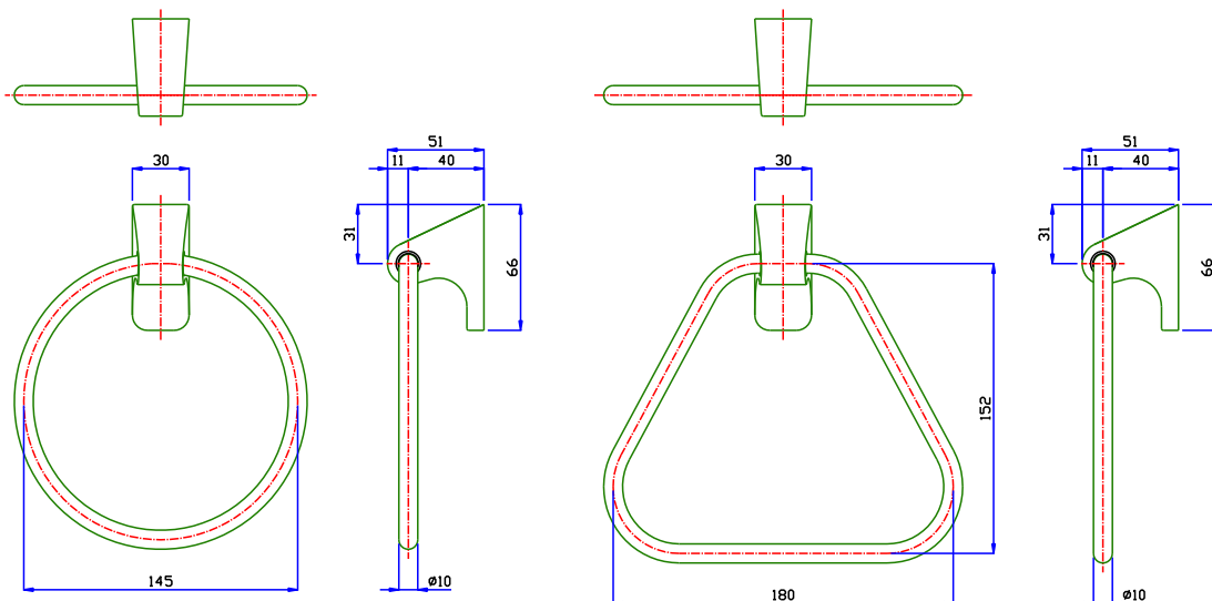
製品寸法図
